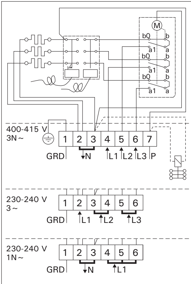
Rys. 10. Schemat elektryczny (3) Obrazek 10. Zapojení topného tělesa 3
