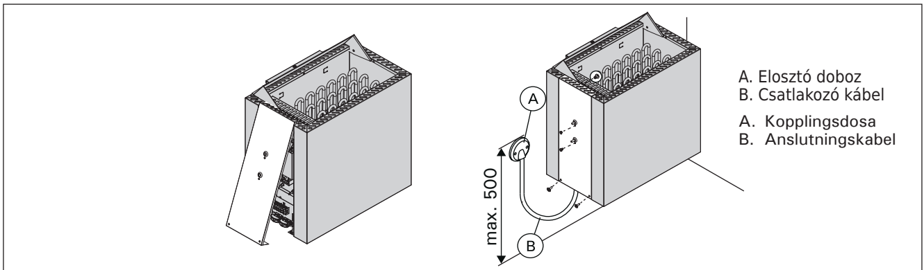
8. ábra. A csatlakozó doboz burkolatának lezárása (minden méret milliméterben értendő) Bild 8. Stänga anslutningshusets front (måttan i millimeter)
