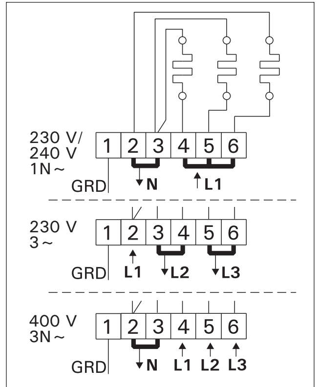
Figura 11. Conexiones eléctricas (3-E) Figura 11. Collegamenti elettrici della stufa 3-E
