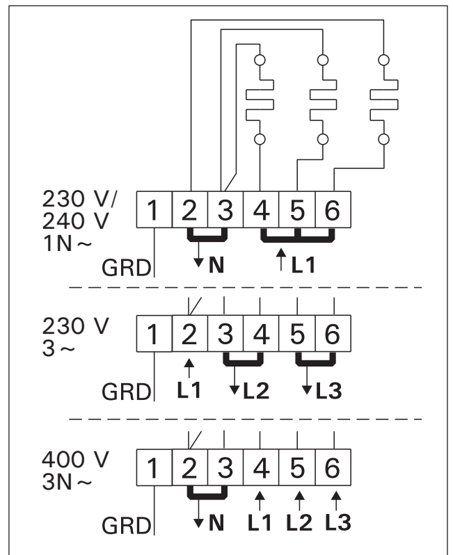
Figura 11. Ligações elétricas do aquecedor 3-E
