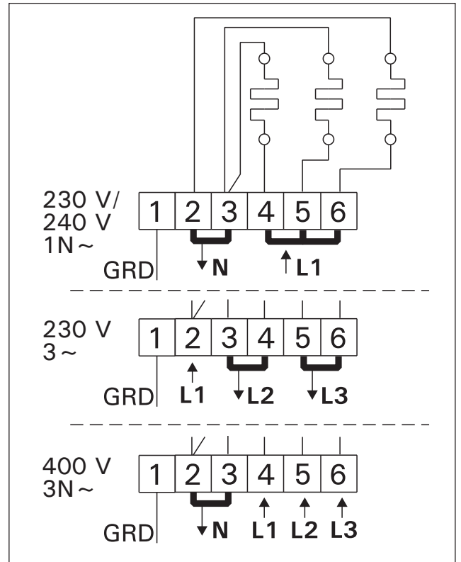
Rys. 11. Schemat elektryczny (3-E) Obrazek 11. Zapojení topného tělesa 3-E
