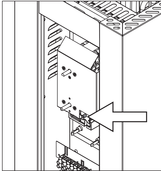
9. ábra A túlmelegedésgátló újraindító gombja Bild 9. Överhettningsskyddets återställningsknapp
