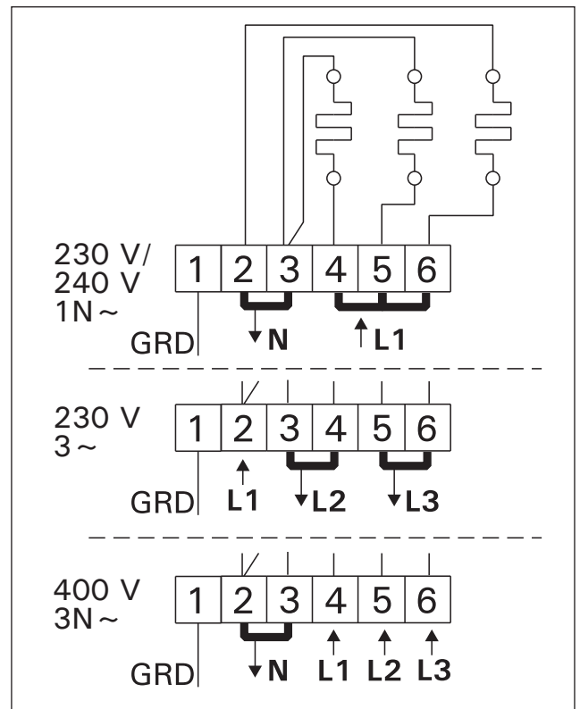
Figure 11. Raccordements électriques du pôle (3-E) Figuur 11. Elektrische aansluitingen (3-E)
